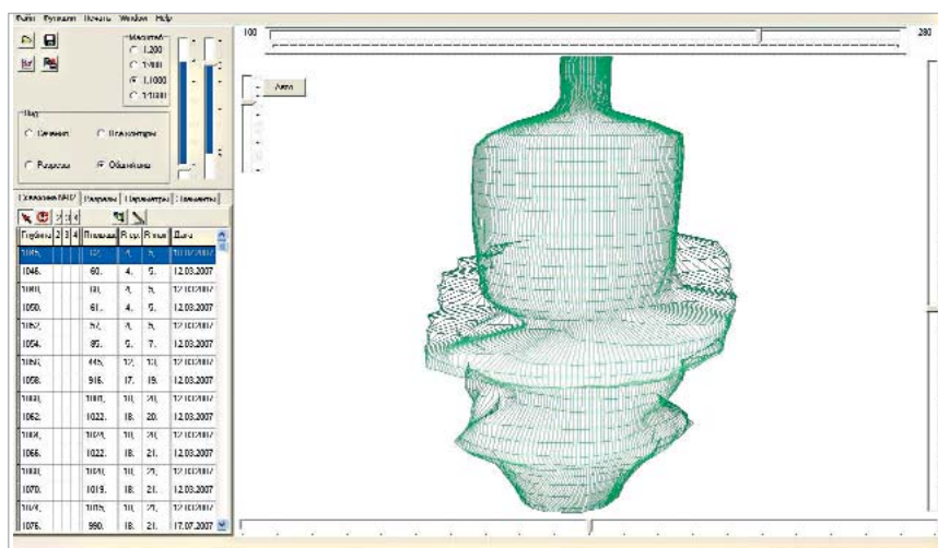
Рис. 3. Обработка результатов эхолотации. Трехмерное изображение размытой полости
