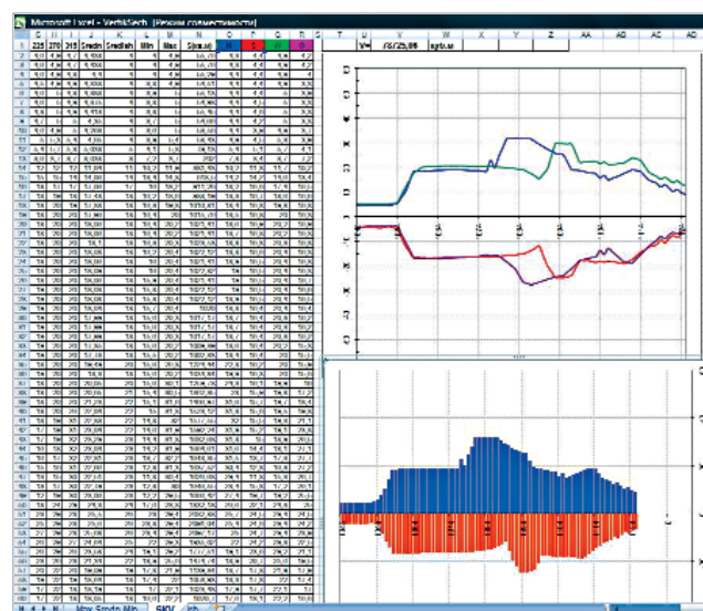
Рис. 5. Обработка результатов эхолотации. Возможность просмотра данных в EXCEL
