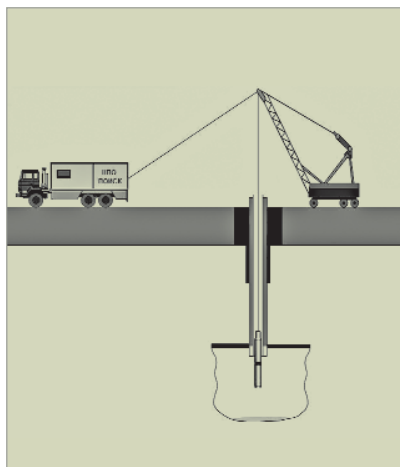
Рис. 2. Схема применения эхолотного комплекса "Сканер-2000"
