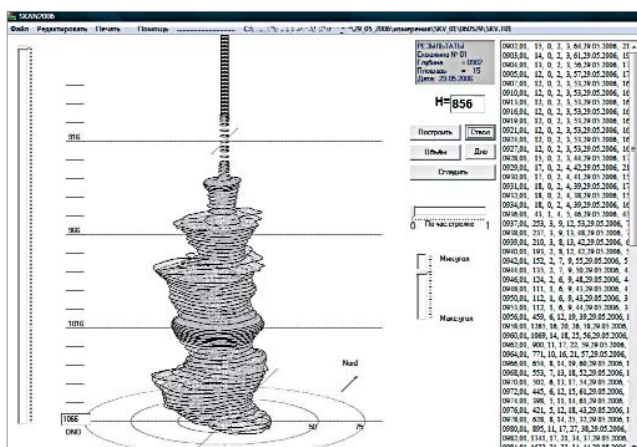
Рис. 4. Обработка результатов эхолотации. Аксонометрическая проекция скважины
